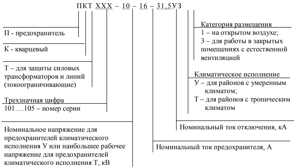
Рис. 5.4. Структура условного обозначения предохранителей
