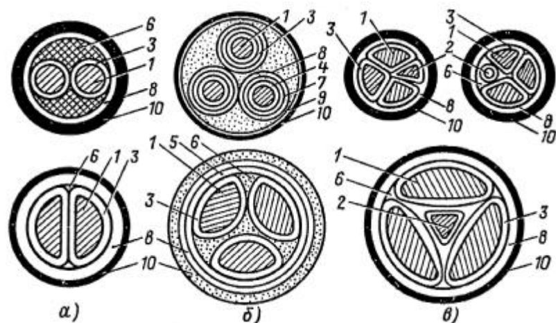
Рис. 2.3. Сечения силовых кабелей:
