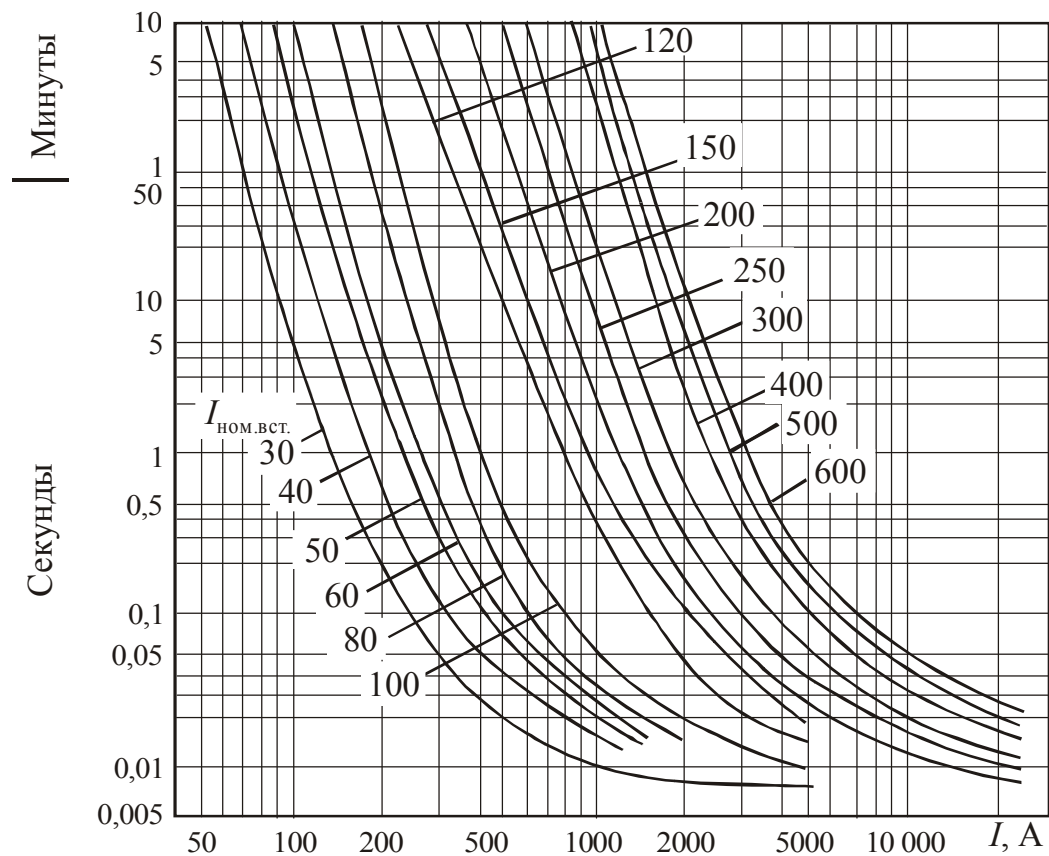
Рис.4.5. Защитные характеристики плавких вставок предохранителей ПН2
