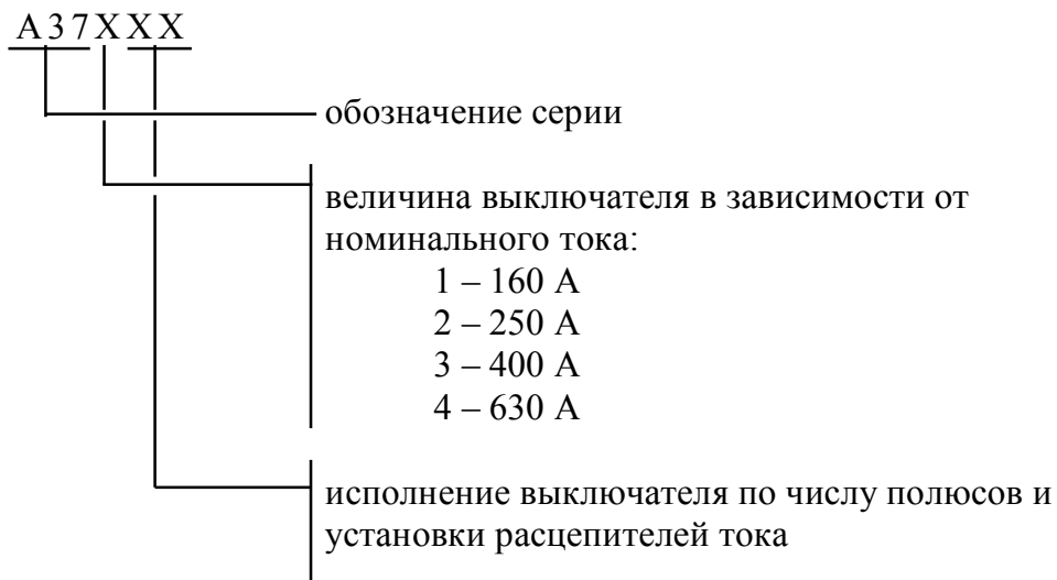
Рис. 4.7. Структура условного обозначения автоматического выключателя серии А3700.
