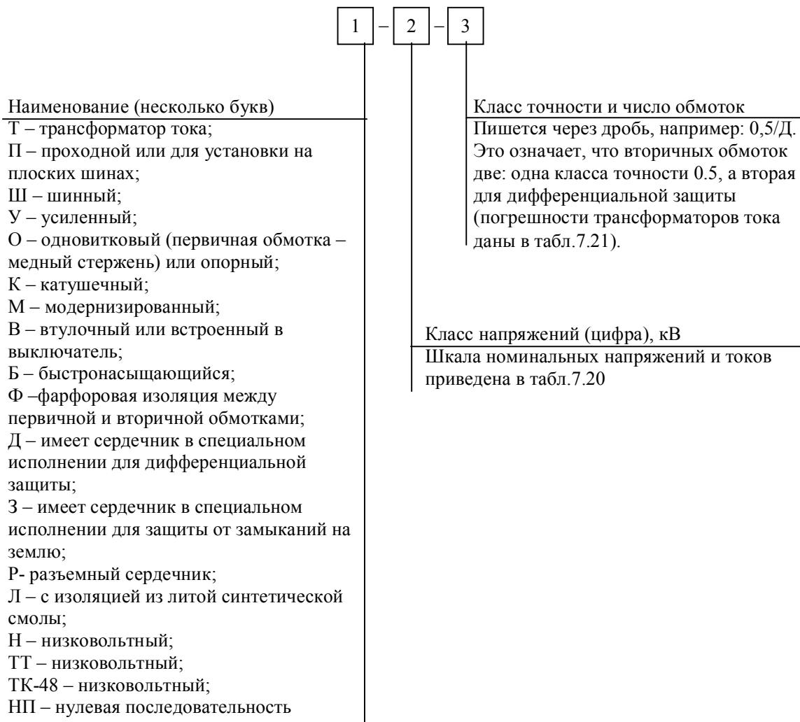
Рис. 5.6. Структура условного обозначения трансформаторов тока
