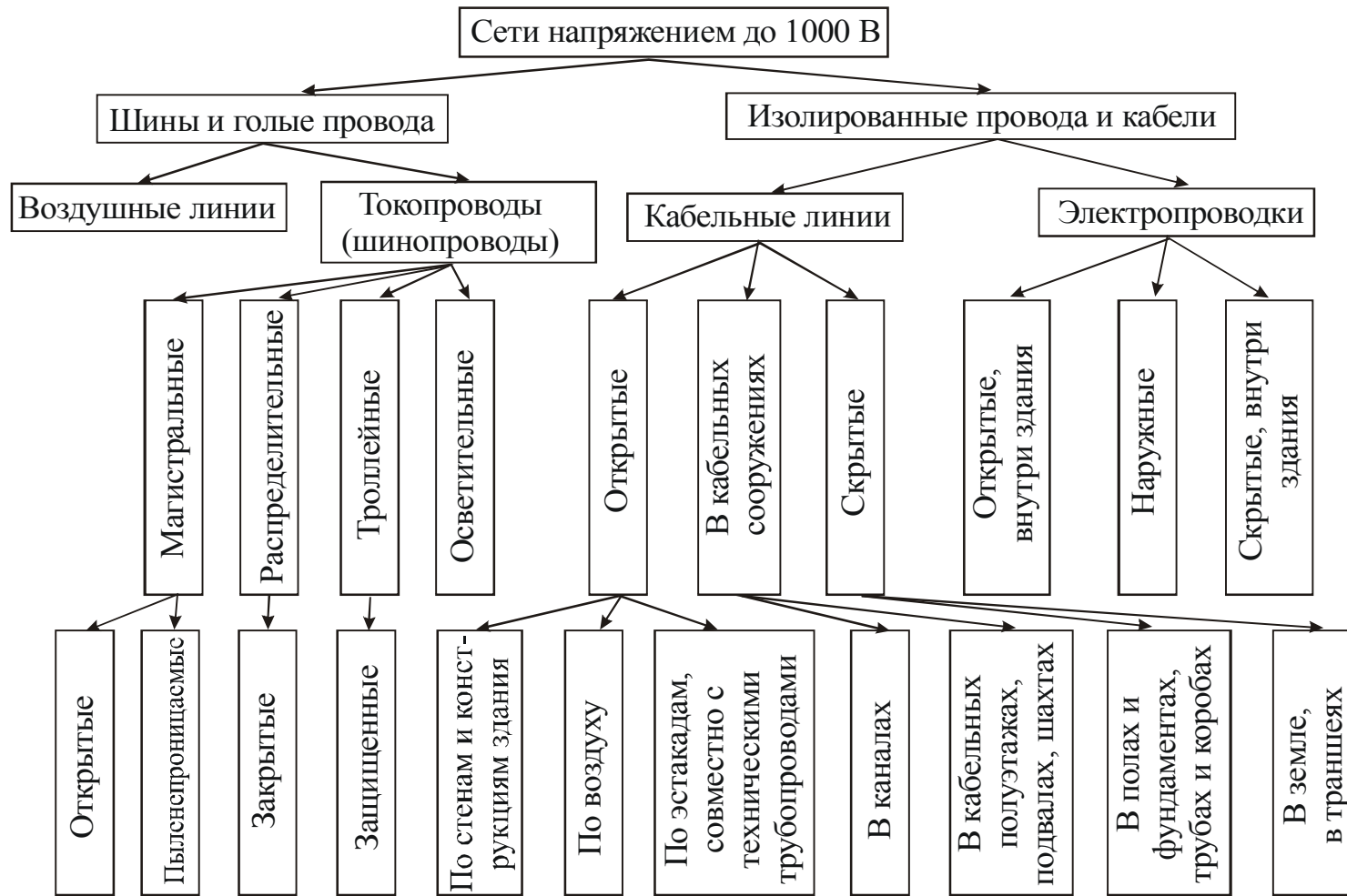
Рис.2.1. Классификация сетей по конструктивным признакам
